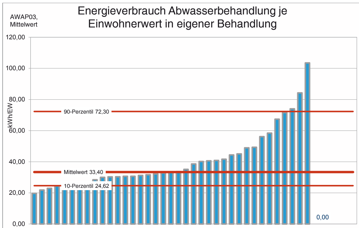
Abbildung 28: Energieverbrauch Abwasserbehandlung
